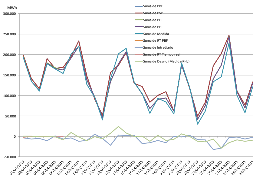
Gráfico 11. Evolución diaria de la transición desde el PBF hasta la producción eólica real. Abril 2015
