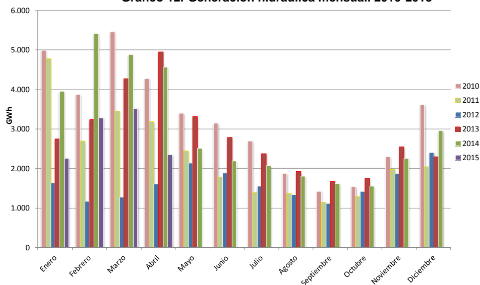
Gráfico 12. Generación hidráulica mensual. 2010-2015
