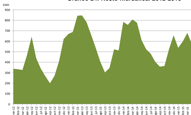
Gráfico 24. Resto hidráulica. 2012-2015
