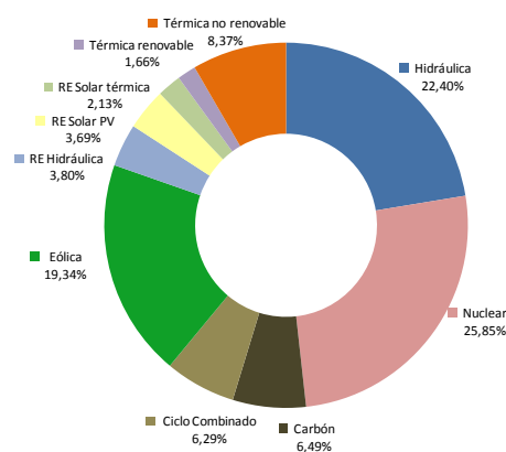
Gráfico 05. Estructura de generación. abril 2014
