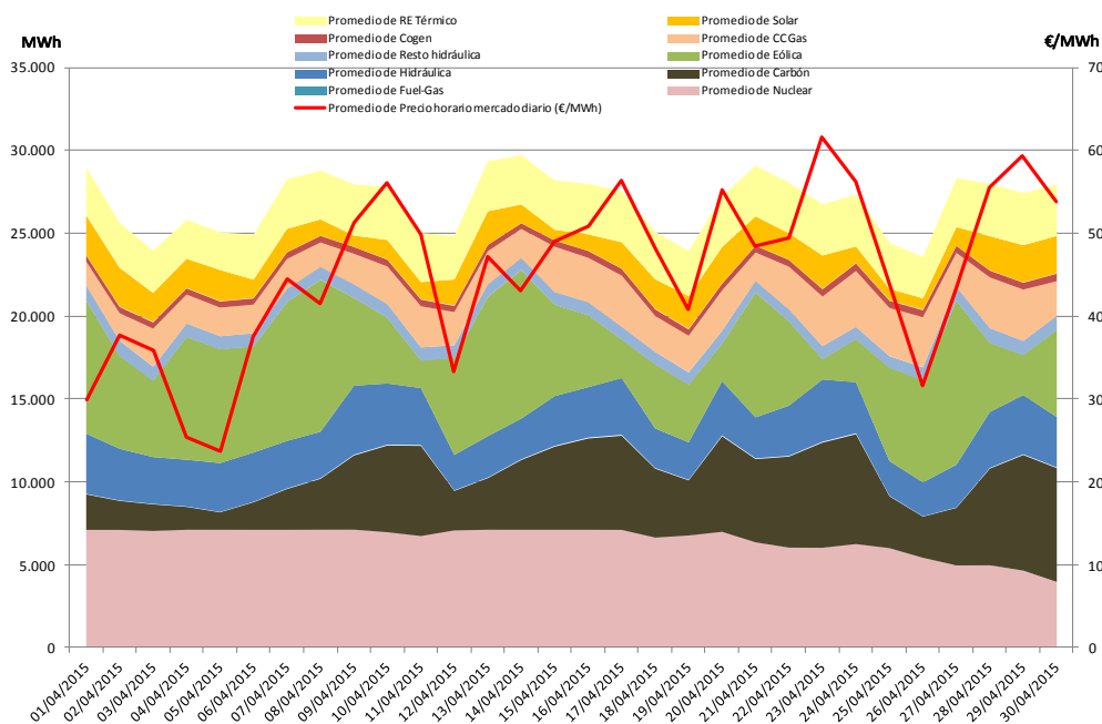
Gráfico 29. Energía por tecnologías y precio medio diario del MD. Abril 2015
