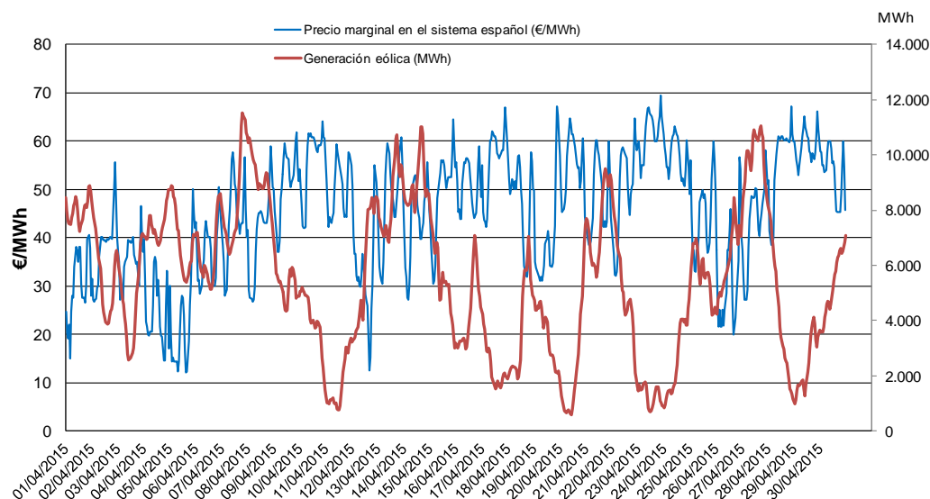
Gráfico 27. Evolución horaria del precio del mercado diario y de la generación eólica. Abril 2014
