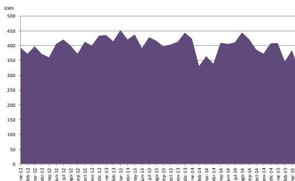
Gráfico 24. Resto hidráulica. 2012-2015
