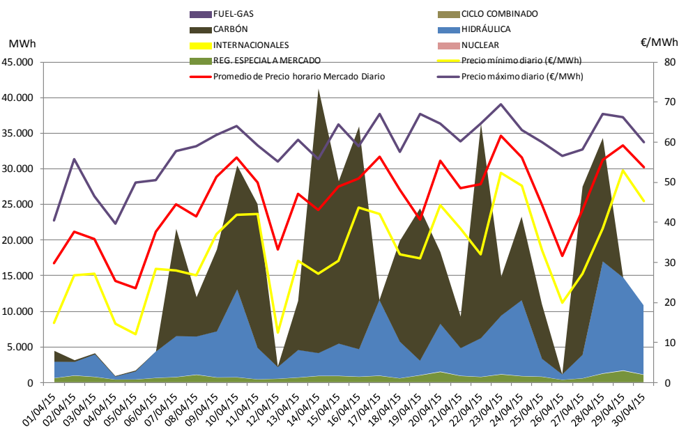
Gráfico 28. Energía por tecnologías casada y ofertada a precio igual o superior al 95% del marginal y precio medio diario del MD. Abril 2015
