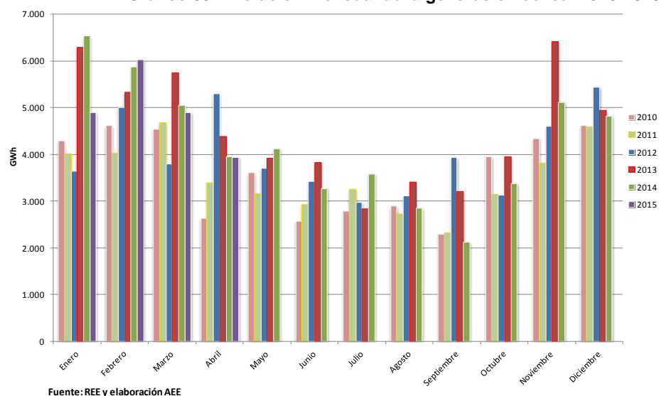
Gráfico 09. Evolución mensual de la generación eólica. 2010-2015
