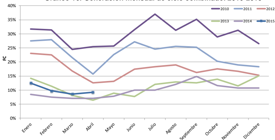
Gráfico 16. Generación mensual de ciclo combinado. 2010-2015
