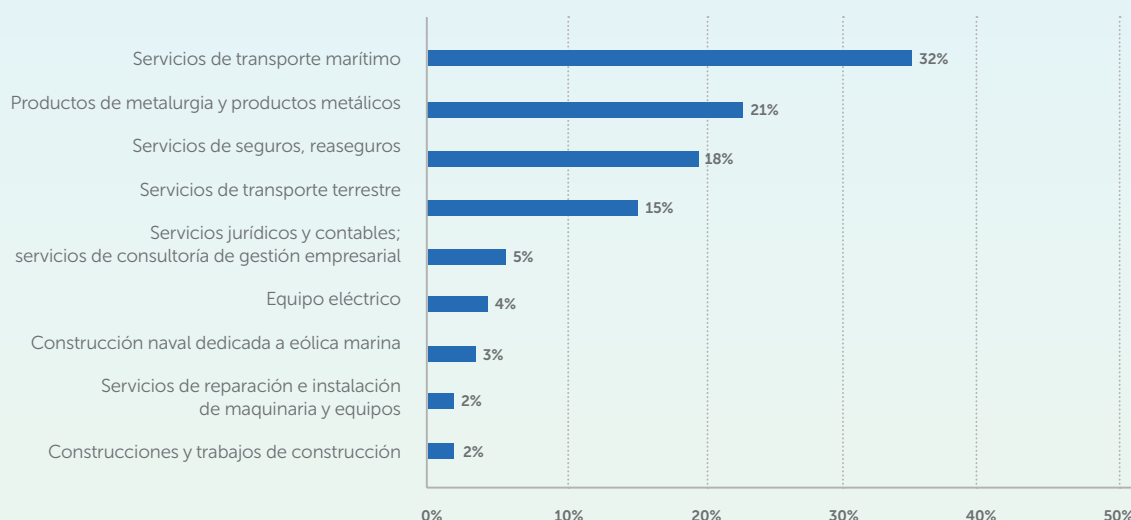
Figura 25. Estructura de demanda indirecta de otros sectores para un parque eólico marino (500 MW)
