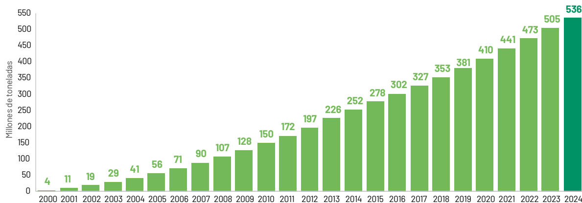
Emisiones de CO 2 evitadas acumuladas 2000-2024
